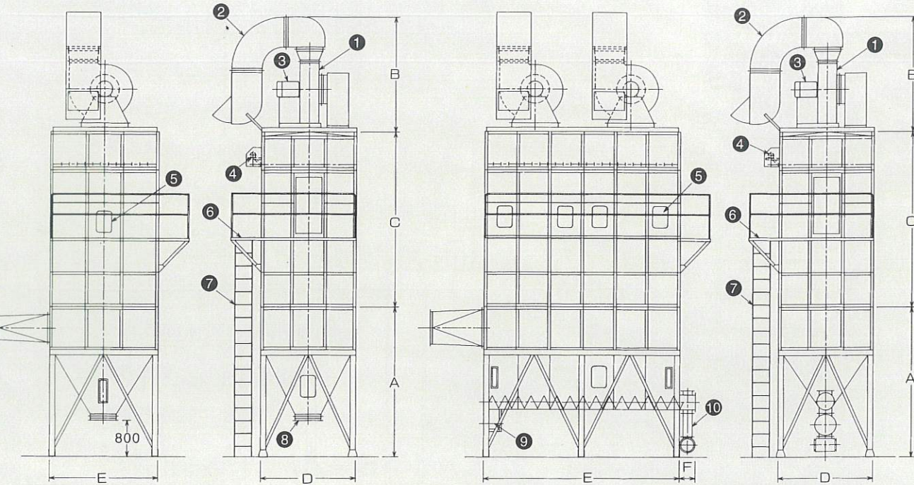
BFH型（下部ホッパー型）
